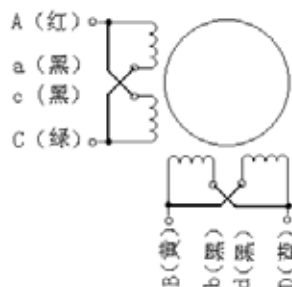
b) 并联接法
